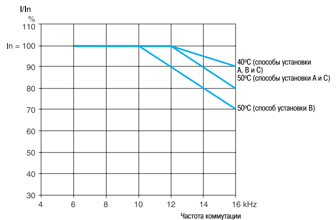
ATV21HU22N4
