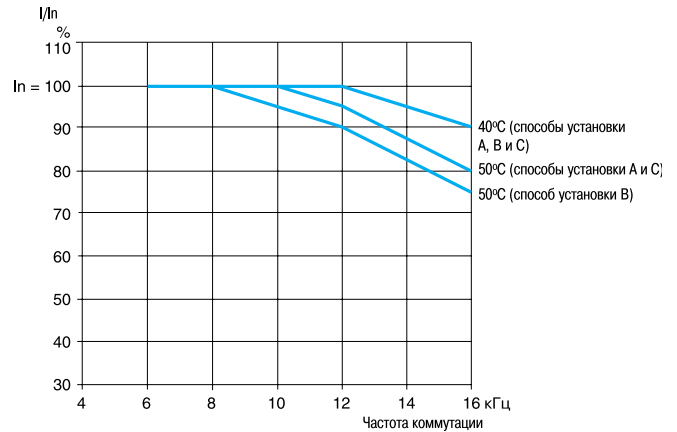
ATV 21HU40M3X
