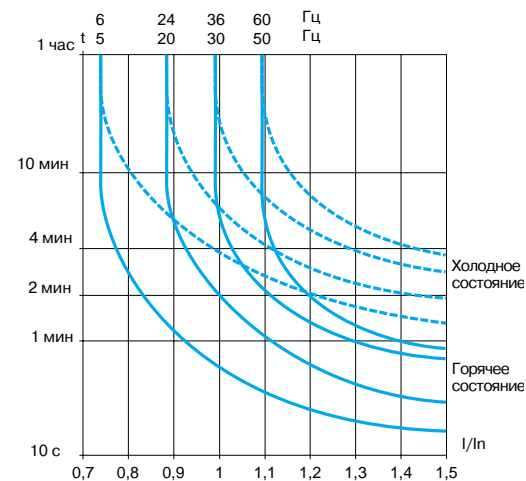
Время-токовые характеристики
