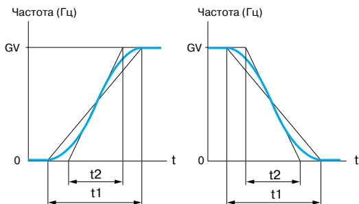
S-образная кривая Фиксированный коэффициент сглаживания с t_2 = 0,6 \times t_1 , где t_1 - настраиваемое время разгона или торможения.
