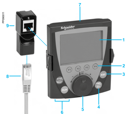
Выносной графический терминал + кабель для удаленного подключения + адаптер RJ45 «гнездо/гнездо»
