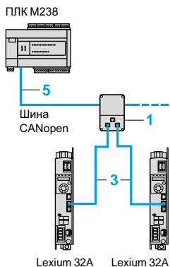
Пример архитектуры с управлением от ПЛК M238
