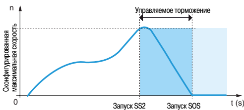
Запуск функции безопасности "Safe Limited Speed" (SLS)
