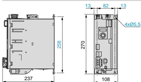
Сервопреобразователи LXM 32D72N4
