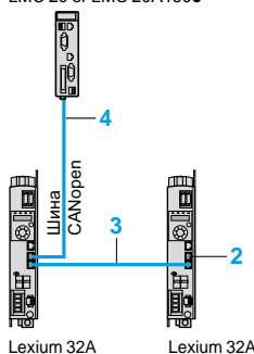
Пример архитектуры с управлением от контроллера перемещения LMC Lexium Controller
