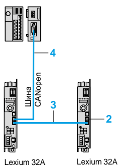
Пример архитектуры с управлением от ПЛК Twido
