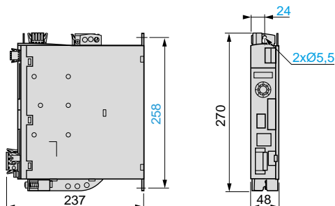
Сервопреобразователи LXM 32MU45M2...MD18N4
