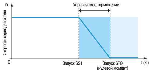
Запуск функции безопасности "Safe Stop 1" (SS1)
