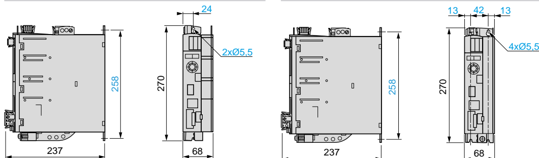
Сервопреобразователи LXM 32D72N4
