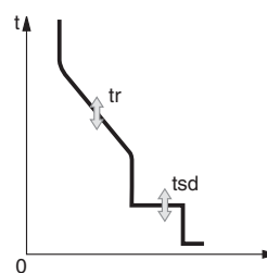
Кривая I^2t OFF
