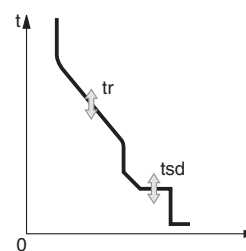
Кривая I^2t ON
