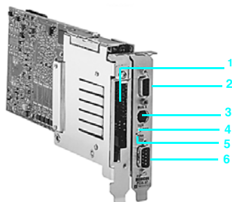
TSX PCI 57 4M
