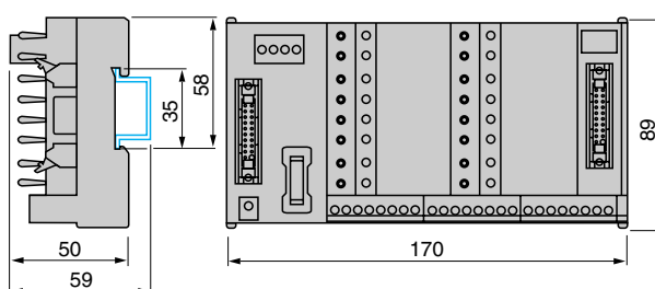
Колodка-эмулятор ABE-7TES160
