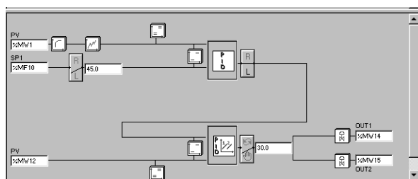
Каскадный контур
