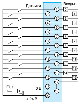
TSX DEY 16D2
