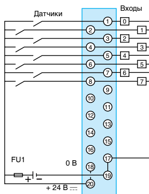
TSX DEY 08D2
