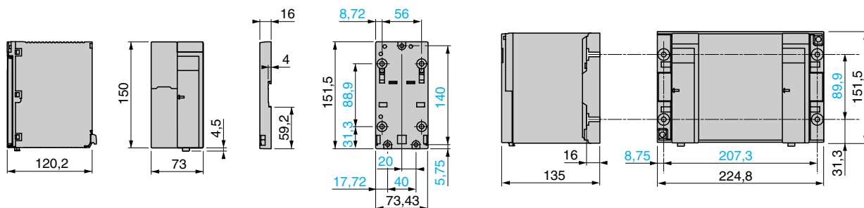
Монтажная пластина (входит в комплект поставки)
