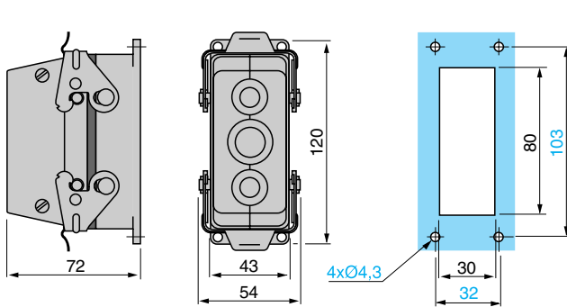
Колodка-эмулятор ABE-7TES160
