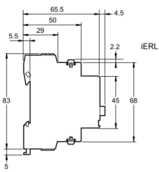
iRLI, iERL
