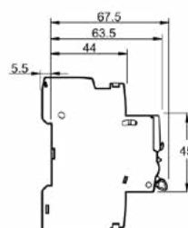
iOF, iSD - 2 to 100 mA - подвійні клемми (A9A26915, A9A26916)
