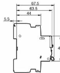
iOF, iSD - подвійні клемми (A9A26905, A9A26906)
