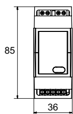
STD400RC/RL
