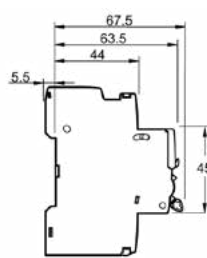
iOF, iSD - подвійні клемми (A9A26905, A9A26906)
