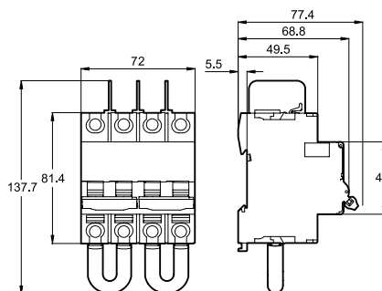
SW60-DC
