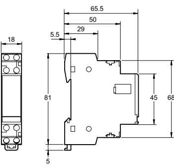
iRBN, iRTBT
