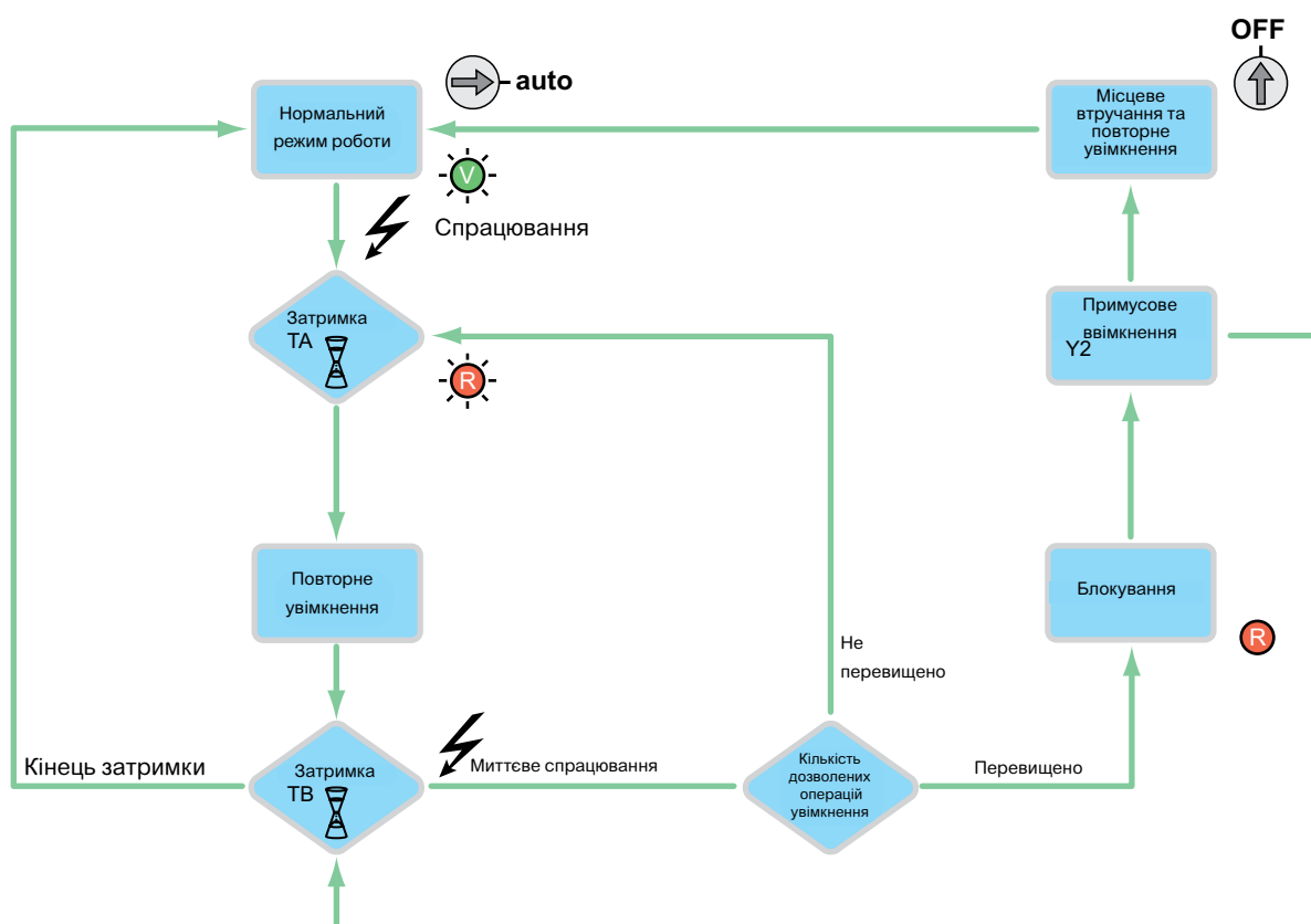
Схема роботи ARA iID
