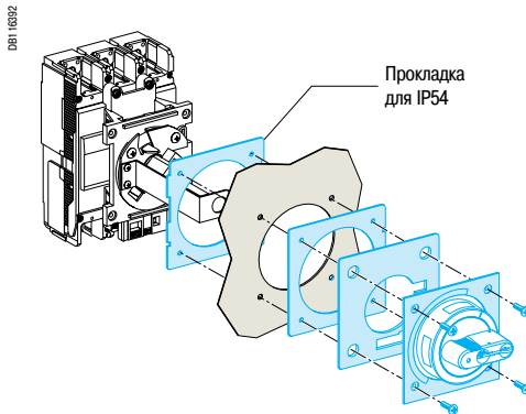
EZC250/EZCV250.
