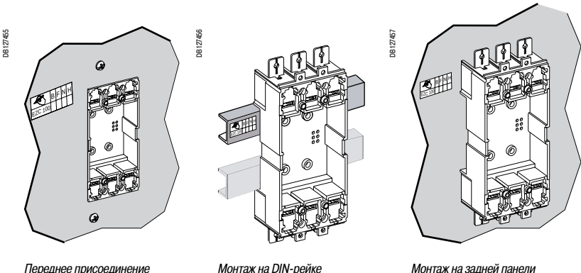
Переднее присоединение
