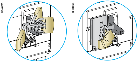
Блокировка рычага управления навесными замками: при помощи съёмного устройства при помощи стационарного устройства
