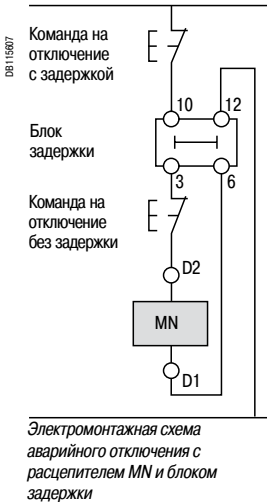
Расцепитель MN с блоком задержки
