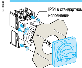
EZC100.
