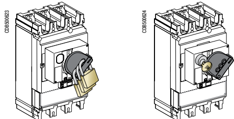
Блокировка поворотной рукоятки навесным или встроенным замком
