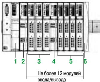
Базовая конфигурация Modicon STB с одним сегментом
