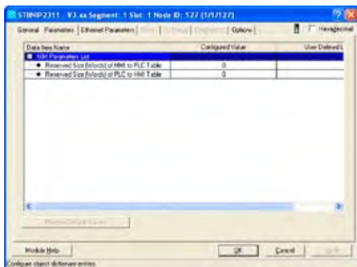
Вкладка «Параметры»: сетевой интерфейсный модуль Ethernet Modbus TCP/IP, два порта STB NIP 231
