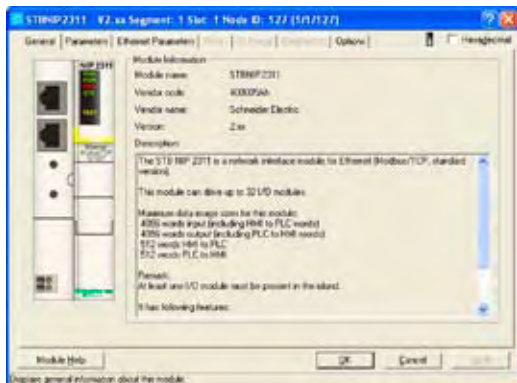
Вкладка «Общие сведения»: сетевой интерфейсный модуль Ethernet Modbus TCP/IP, два порта STB NIP 231
