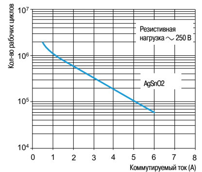
Электрическая износостойкость
