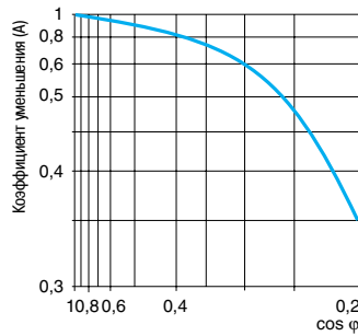
Коэффициент уменьшения для индуктивной нагрузки \sim (в зависимости от коэффициента мощности cos φ)
