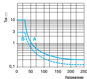
Максимальная коммутационная способность с резистивной нагрузкой \text{---}
