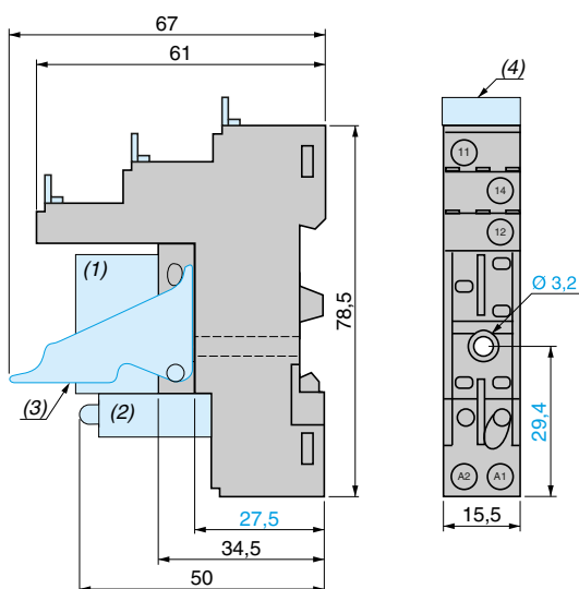
(1) Реле. (2) Модуль защиты. (3) Скоба-держатель. (4) Этикетка.
