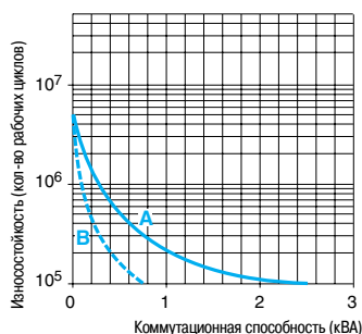
Электрическая износостойкость контактов Резистивная нагрузка \sim
